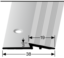
330 versenkt gebohrt countersunk drilled à percement noyé
