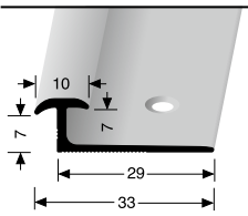
297 versenkt gebohrt countersunk drilled à percement noyé
