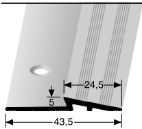
332 versenkt gebohrt countersunk drilled à percement noyé
