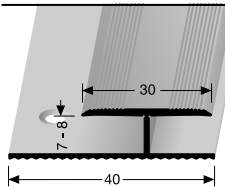
221 ♦ versenkt gebohrt countersunk drilled à percement noyé
