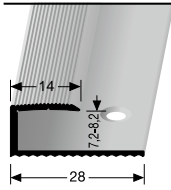
210 versenkt gebohrt countersunk drilled à percement noyé
