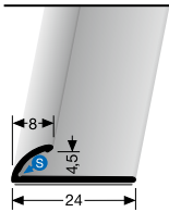
380 SK selbstklebend self-adhesive auto-adhésif
