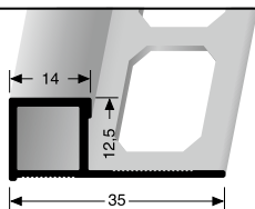
CT125 G \updownarrow 12,5 mm geschlossen gestanzt punched base estampé fermé
