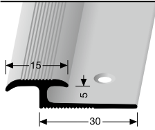
292 versenkt gebohrt countersunk drilled à percement noyé
