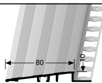
PR100 G \updownarrow 10 mm geschlossen gestanzt punched base estampé fermé
