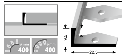
303 ⇄ 8 mm offen gestanzt open punched estampé ouvert
