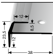
857 versenkt gebohrt countersunk drilled à percement noyé
