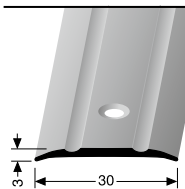
439 mittig versenkt gebohrt centrally countersunk drilled à percement noyé central
