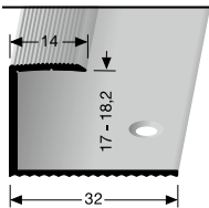
217 versenkt gebohrt countersunk drilled à percement noyé
