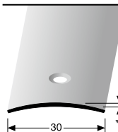
451 mittig versenkt gebohrt centrally countersunk drilled à perçement noyé central
