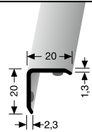
271 SK selbstklebend self-adhesive auto-adhésif
