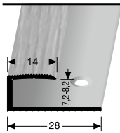
210 H mit Holzdekor with wood decor avec décor bois
