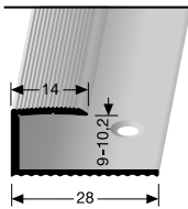
212 versenkt gebohrt countersunk drilled à percement noyé
