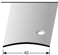
454 S seitlich versenkt gebohrt laterally countersunk drilled à perçement noyé latéral
