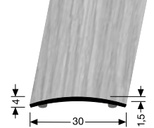
459 H/SK mit Holzdekor, selbstklebend with wood decor, self-adhesive avec décor bois, auto-adhésif
