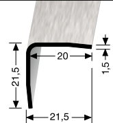
272 U ungebohrt, 3-fach gekantet undrilled, 3-side edged non percé, 3 fois plié
