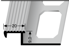
TR090 G \updownarrow 9 mm geschlossen gestanzt punched base estampé fermé
