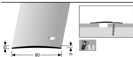
465 S seitlich versenkt gebohrt laterally countersunk drilled à perçement noyé latéral
