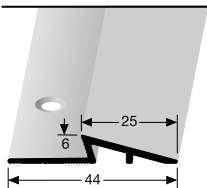
333 versenkt gebohrt countersunk drilled à percement noyé
