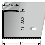
219 ♦ versenkt gebohrt countersunk drilled à percement noyé
