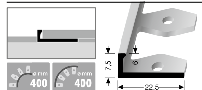
307 ⇄ 6 mm offen gestanzt open punched estampé ouvert
