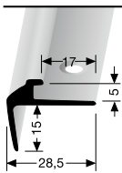
850 versenkt gebohrt countersunk drilled à percement noyé
