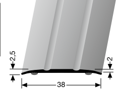
438 SK selbstklebend self-adhesive auto-adhésif
