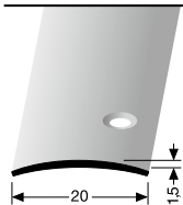
472 S seitlich versenkt gebohrt laterally countersunk drilled à perçement noyé latéral
