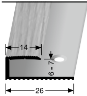
211 H mit Holzdekor with wood decor avec décor bois
