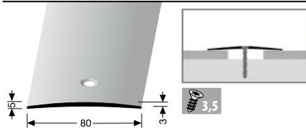
465 mittig versenkt gebohrt centrally countersunk drilled à perçement noyé central
