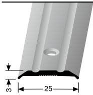
230 mittig versenkt gebohrt centrally countersunk drilled à percement noyé central
