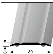
439 SK selbstklebend self-adhesive auto-adhésif
