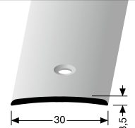
456 mittig versenkt gebohrt centrally countersunk drilled à percement noyé central
