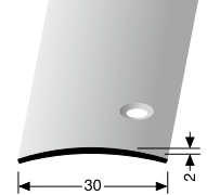
473 S seitlich versenkt gebohrt laterally countersunk drilled à percement noyé latéral
