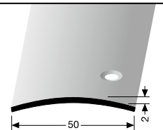
475 S seitlich versenkt gebohrt laterally countersunk drilled à percement noyé latéral
