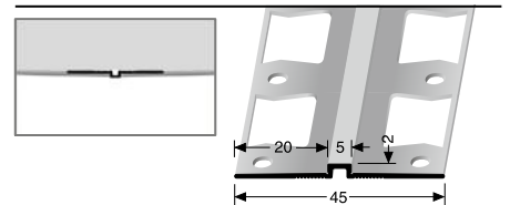
170 G geschlossen gestanzt punched base estampé fermé
