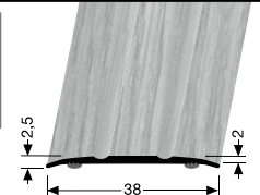
438 H/SK mit Holzdekor, selbstklebend with wood decor, self-adhesive avec décor bois, auto-adhésif
