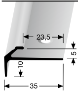
855 versenkt gebohrt countersunk drilled à percement noyé
