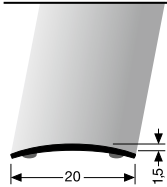
472 SK selbstklebend self-adhesive auto-adhésif
