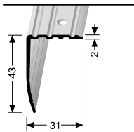
540 versenkt gebohrt countersunk drilled à percement noyé
