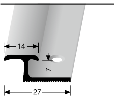
223 ♦ versenkt gebohrt countersunk drilled à percement noyé
