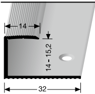
215 versenkt gebohrt countersunk drilled à percement noyé
