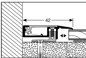
550 \updownarrow 7 - 16 mm \blacklozenge versenkt gebohrt countersunk drilled à perçement noyé
