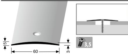
464 mittig versenkt gebohrt centrally countersunk drilled à perçement noyé central
