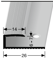
211 versenkt gebohrt countersunk drilled à percement noyé
