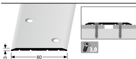
446 versetzt versenkt gebohrt offset countersunk drilled à perçement noyé décalé
