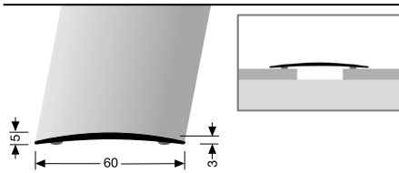
464 SK selbstklebend self-adhesive auto-adhésif
