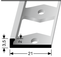
299 G geschlossen gestanz punched base estampé fermé
