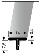
290 U F8 ungebohrt, nicht biegbar undrilled, not bendable non percé, non déformable
