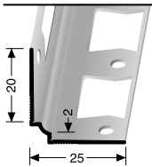
160 G geschlossen gestanz punched base estampé fermé
