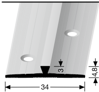
365 versetzt versenkt gebohrt offset countersunk drilled à perçement noyé décalé
