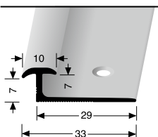
297 R versenkt gebohrt, Revisionsrahmen - verschweißt countersunk drilled, Floor access cover frame - welded à percement noyé, cadre de révision pour sol - soudé
