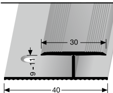
222 ♦ versenkt gebohrt countersunk drilled à percement noyé
