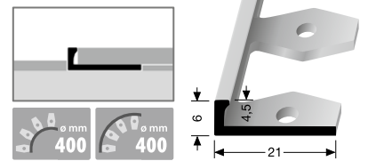
302 ⇄ 4,5 mm offen gestanzt open punched estampé ouvert
