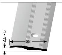
364 versenkt gebohrt countersunk drilled à percement noyé
