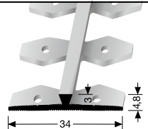
365 EB ⇄ 3 mm offen gestanzt open punched estampé ouvert
