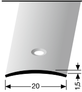
472 mittig versenkt gebohrt centrally countersunk drilled à perçement noyé central
