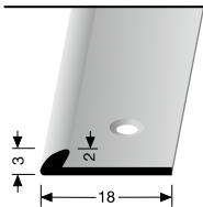
355 versenkt gebohrt countersunk drilled à perçement noyé
