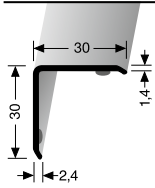
273 SK selbstklebend self-adhesive auto-adhésif
