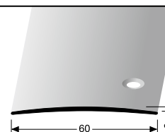
167 S seitlich versenkt gebohrt laterally countersunk drilled à percement noyé latéral
