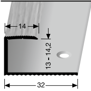
214 H mit Holzdekor with wood decor avec décor bois
