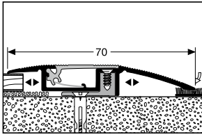
552 \updownarrow 7 - 16 mm \blacklozenge versenkt gebohrt countersunk drilled à perçement noyé
