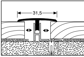
561 H \updownarrow 12 - 17 mm mit Holzdekor with wood decor avec décor bois
