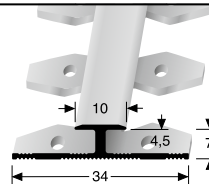
368 EB ⇄ 4,5 mm offen gestanzt open punched estampé ouvert
