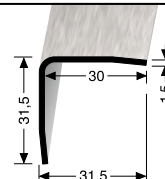
274 U ungebohrt, 3-fach gekantet undrilled, 3-side edged non percé, 3 fois plié
