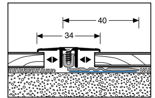
288 SK \updownarrow 6,5 – 16 mm*
