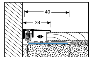
287 N/SK \updownarrow 6,5 – 16 mm*
