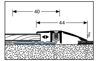
286 SK \updownarrow 6,5 – 16 mm*
