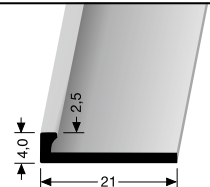
300 U \hat{=} 2,5 mm ungestanzt unpunched non estampé
