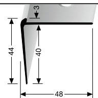
862 EC-L versenkt gebohrt countersunk drilled à perçement noyé
