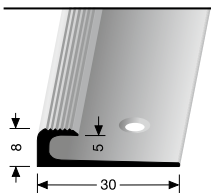
806 versenkt gebohrt countersunk drilled à percement noyé
