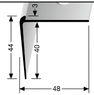
862 EC versenkt gebohrt countersunk drilled à perçement noyé
