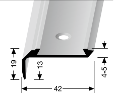
701 versenkt gebohrt countersunk drilled à perçement noyé
