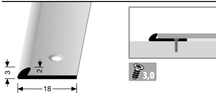
355 versenkt gebohrt countersunk drilled à percement noyé
