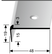
860 EC-R versenkt gebohrt countersunk drilled à perçement noyé
