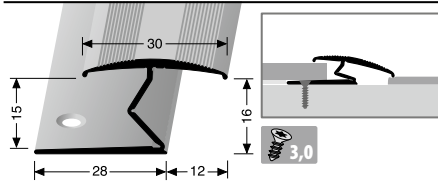
383 versenkt gebohrt countersunk drilled à percement noyé
