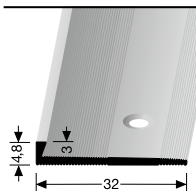
364 versenkt gebohrt countersunk drilled à percement noyé
