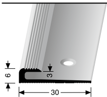
804 versenkt gebohrt countersunk drilled à percement noyé
