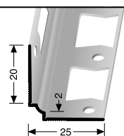
160 G geschlossen gestanz perforated anchor estampé fermé
