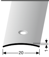
471 mittig versenkt gebohrt centrally countersunk drilled à perçement noyé central
