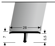
293 einfach biegbar easy bendable cintrable
