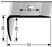
712 T versenkt gebohrt countersunk drilled à perçement noyé
