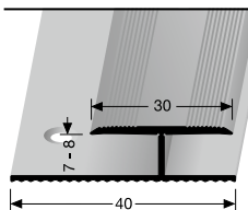
221 ♦ versenkt gebohrt countersunk drilled à percement noyé
