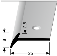
341 versenkt gebohrt countersunk drilled à percement noyé
