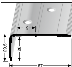
715 versetzt versenkt gebohrt, für zwei Einlagen offset countersunk drilled, for two inserts à perçement noyé décalé, pour deux inserts
