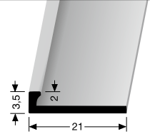
299 U \hat{=} 2 mm ungestanzt unpunched non estampé
