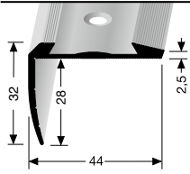
705 versenkt gebohrt countersunk drilled à perçement noyé
