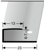
011 versenkt gebohrt countersunk drilled à percement noyé
