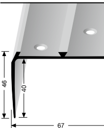
704 versetzt versenkt gebohrt offset countersunk drilled à perçement noyé décalé
