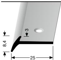
342 versenkt gebohrt countersunk drilled à percement noyé
