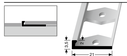
299 G geschlossen gestanz perforated anchor estampé fermé
