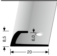
362 versenkt gebohrt countersunk drilled à percement noyé
