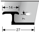
223 ♦ versenkt gebohrt countersunk drilled à percement noyé
