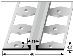
301 S \updownarrow 3 mm
