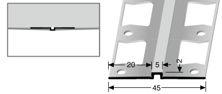
170 G geschlossen gestanz perforated anchor estampé fermé
