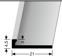
301 U \hat{=} 3 mm ungestanzt unpunched non estampé
