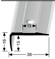
711 T versenkt gebohrt countersunk drilled à perçement noyé
