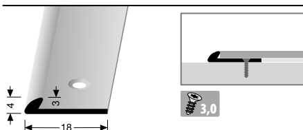
357 versenkt gebohrt countersunk drilled à percement noyé
