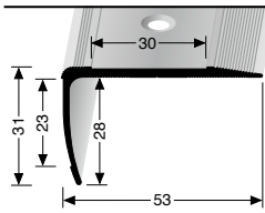
713 versenkt gebohrt, für zwei Einlagen countersunk drilled, for two inserts à perçement noyé, pour deux inserts
