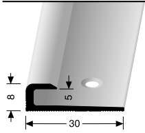
802 versenkt gebohrt countersunk drilled à percement noyé
