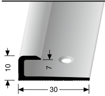
803 versenkt gebohrt countersunk drilled à percement noyé
