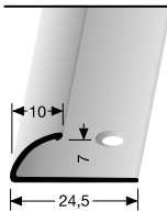
390 versenkt gebohrt countersunk drilled à percement noyé
