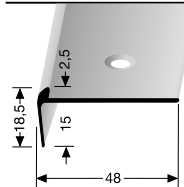
859 EC-R versenkt gebohrt countersunk drilled à perçement noyé
