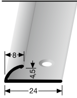
380 versenkt gebohrt countersunk drilled à percement noyé
