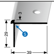
871 EV-L versenkt gebohrt, zweiteilig countersunk drilled, two-part à perçement noyé, en deux parties
