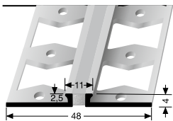
300 S \updownarrow 2,5 mm
