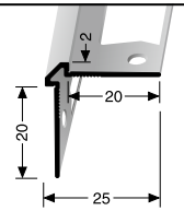
155 G geschlossen gestanz perforated anchor estampé fermé
