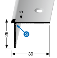
871 EC versenkt gebohrt countersunk drilled à perçement noyé
