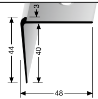
862 EC-R versenkt gebohrt countersunk drilled à perçement noyé
