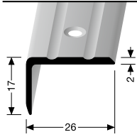
237 versenkt gebohrt countersunk drilled à perçement noyé
