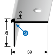
871 EC-L versenkt gebohrt countersunk drilled à perçement noyé
