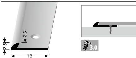
356 versenkt gebohrt countersunk drilled à percement noyé
