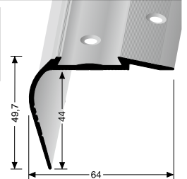
707 C versetzt versenkt gebohrt offset countersunk drilled à perçement noyé décalé
