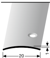
471 S seitlich versenkt gebohrt laterally countersunk drilled à perçement noyé latéral
