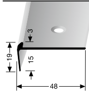
860 EC versenkt gebohrt countersunk drilled à perçement noyé
