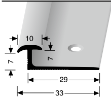
297 versenkt gebohrt countersunk drilled à percement noyé
