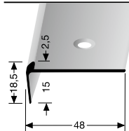
859 EC-L versenkt gebohrt countersunk drilled à perçement noyé
