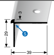
871 EV-R versenkt gebohrt, zweiteilig countersunk drilled, two-part à perçement noyé, en deux parties
