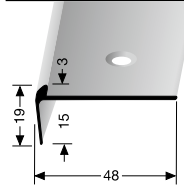
860 EC-L versenkt gebohrt countersunk drilled à perçement noyé
