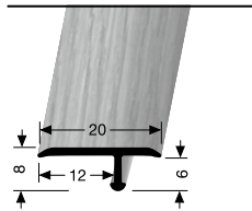
291 H einfach biegbar, mit Holzdekor easy bendable, with wood decor cintrable, avec bande décorative
