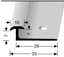
297 R versenkt gebohrt, Revisionsrahmen - verschweißt countersunk drilled, Floor access cover frame - welded à percement noyé, cadre de révision pour sol - soudé
