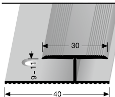
222 versenkt gebohrt countersunk drilled à percement noyé
