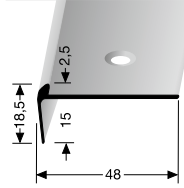
859 EC versenkt gebohrt countersunk drilled à perçement noyé
