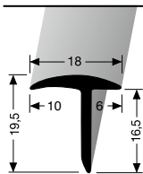
294 versenkt gebohrt countersunk drilled à percement noyé
