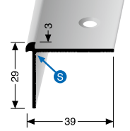
871 EC-R versenkt gebohrt countersunk drilled à perçement noyé
