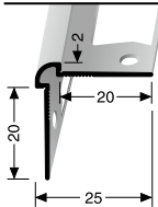
150 G geschlossen gestanzt perforeated anchor estampé fermé
