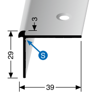
871 EV versenkt gebohrt, zweiteilig countersunk drilled, two-part à perçement noyé, en deux parties
