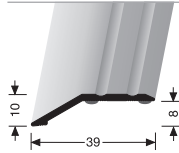
244 SK SEUIL D'ADAPTATION AANPASSINGSPROFIEL
