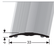
231 SK SEUIL DE RACCORDEMENT VERBINDINGSPROFIEL
