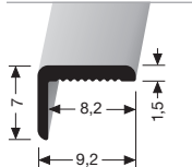
279 U BORD D'ANGLE HOEKRAND
