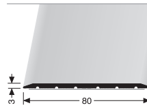
444 SK SEUIL DE RACCORDEMENT VERBINDINGSPROFIEL
