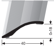
247 SK SEUIL D'ADAPTATION AANPASSINGSPROFIEL
