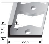
307 G BORDURE PERFORÉE GEPERFOREERDE RANDAFWERKING
