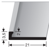
299 U SEUIL D'ARRÊT RANDPROFIEL
