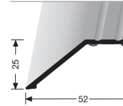
245 SK SEUIL D'ADAPTATION AANPASSINGSPROFIEL
