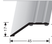
241 SK SEUIL D'ADAPTATION AANPASSINGSPROFIEL
