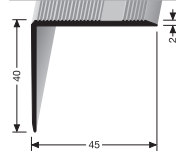
229 U BORD D'ANGLE HOEKRAND
