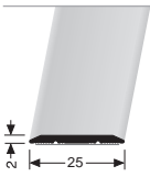
442 SK SEUIL DE RACCORDEMENT VERBINDINGSPROFIEL
