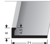
302 U SEUIL D'ARRÊT RANDPROFIEL
