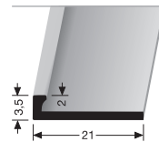
299 U SEUIL D'ARRÊT RANDPROFIEL
