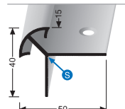
879 BORD D'ANGLE HOEKRAND
