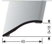
248 SK SEUIL D'ADAPTATION AANPASSINGSPROFIEL
